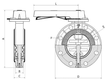
Затвор дисковый ХПВХ с рукояткой EPDM Comer d110 (DN90)
