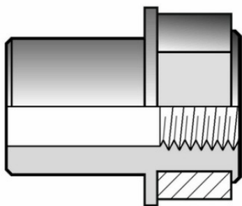
Адаптер с внутренней резьбой PP-H FIP 50x1 1/4 SDR11 PN6
