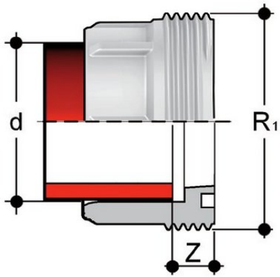
Муфтовая вставка ПВДФ d40 SDR21 PN16
