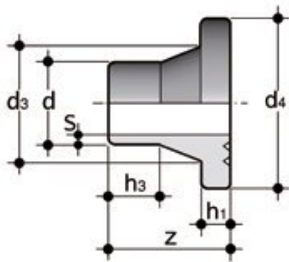
Бурт под фланец для стыковой сварки PP-H FIP (PN6) d500 SDR17.6 PN6
