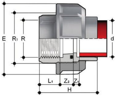
Разборная муфта с ВР, раструбная сварка PP-H (FKM) FIP 32x1 PN10
