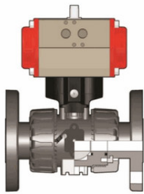
Шаровой кран промышленного применения VKD ПВХ с пневмоприводом, EPDM, FIP d20 (DN15)
