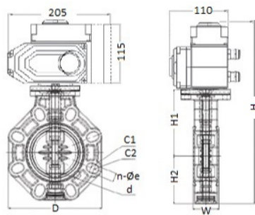
Дисковый затвор IFK PP-H с электрическим приводом 220V AC, EPDM, IPS d225 (DN200)
