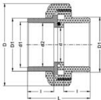
Муфта разборная для раструбной сварки PP-H IPS (EPDM) d90 PN10
