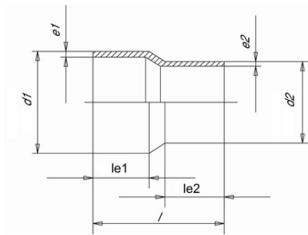
Муфта редукционная ПВДФ (Simona) 225x200 SDR33 PN10
