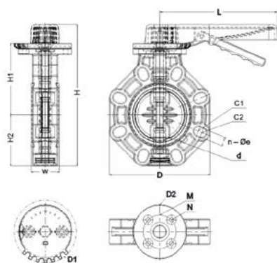
Затвор дисковый ХПВХ с рукояткой EPDM IPS d160 (DN150)
