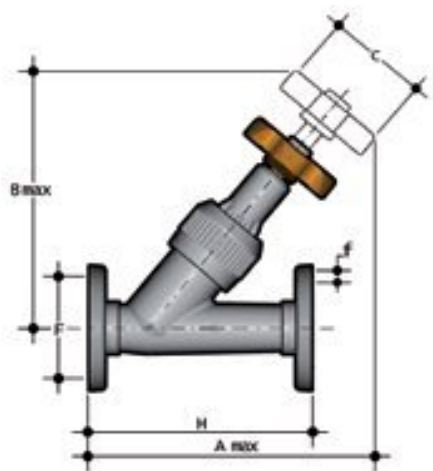
Угловой вентиль VVOV PBX с фланцевыми окончаниями, EPDM, FIP d63 (DN50)
