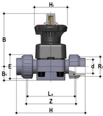
Мембранный клапан DKLUIV ПВХ с разборными муфтовыми окончаниями, EPDM, FIP d63 (DN50)
