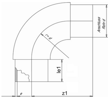
Изгиб 90° PP-H Simona (PN6) d63 SDR17.6 PN6
