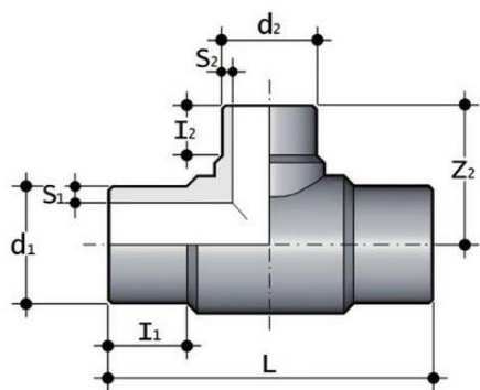
Тройник редукционный для стыковой сварки PP-H FIP 200x160 SDR17.6 PN10
