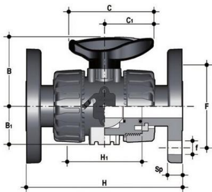
Шаровой кран VKD ПВДФ с фланцевыми окончаниями d50 (DN40)
