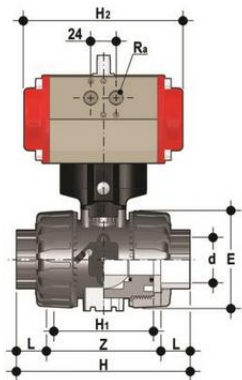
Шаровой кран VKD ХПВХ с пневмоприводом НЗ с муфтовыми окончаниями d50 (DN40)
