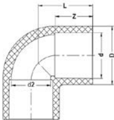
Отвод 90° ХПВХ IPS (Model B) d450 PN10
