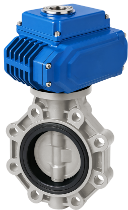
Дисковый затвор IFK PP-H с электрическим приводом 24V DC, EPDM, IPS d110 (DN100)
