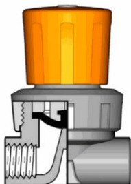
Мембранный мини-клапан VMFV ПБХ с муфтовыми окончаниями с ВР, EPDM, FIP R1/4" (DN8)
