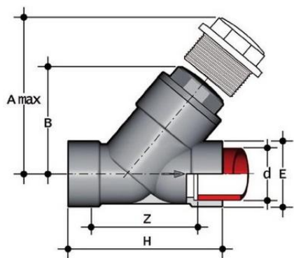
Угловой обратный клапан VR с муфтовыми окончаниями, (уплотнение EPDM) PP-H d90
