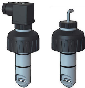
Стандартный датчик расхода с крыльчатым колесом, датчик Холла
