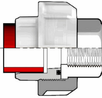
Муфта переходная разборная НР ПВДФ 25x3/4 SDR21 PN16
