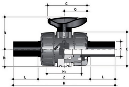
Шаровой кран ПВХ промышленного применения VKD с патрубками из ПЭ (CVDE), EPDM, FIP d25 (DN20)
