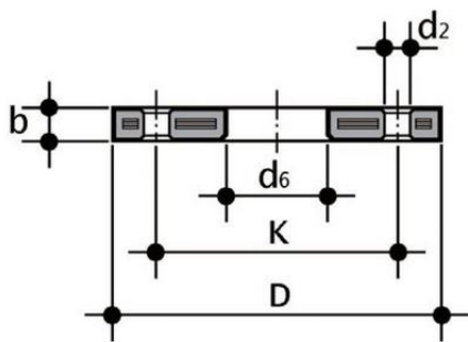
Свободный фланец PP-H FIP d630 PN10
