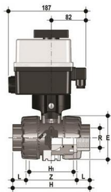
Шаровой кран VKD с эл.приводом 90-240V, резьбовые окончания (уплотнение EPDM) PP-H R1/2" (DN15)
