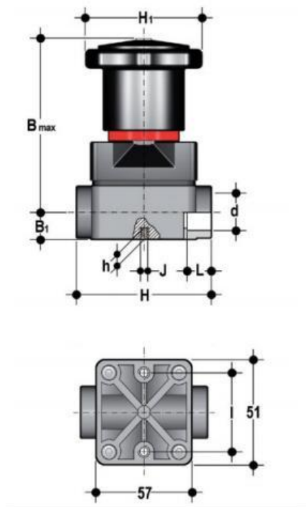
Компактный мембранный клапан CMIV PBX с муфтовыми окончаниями, PTFE, FIP d20 (DN15)
