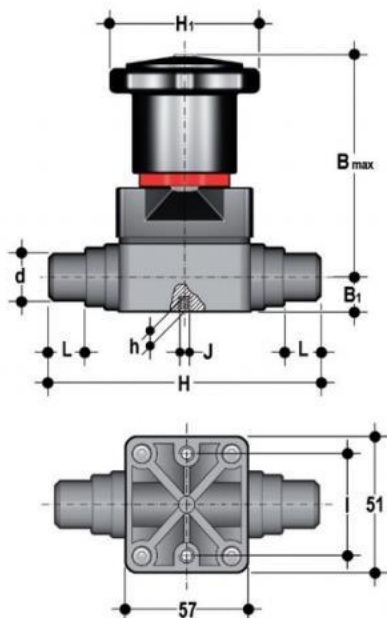
Компактный мембранный клапан ПВХ с пневмоприводом, CM, FKM, FIP d20 (DN15)
