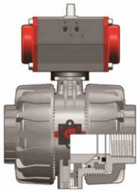
Шаровой кран VKD ПВХ с пневмоприводом ДвД с резьбовыми окончаниями, EPDM, FIP R3" (DN80)
