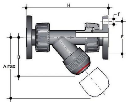
Грязевой фильтр RVUOM с фланцевыми окончаниями (уплотнение FKM) PP-H d40 (DN32)
