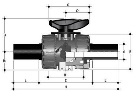
Шаровой кран для регулирования потока VKR с партрубками из ПЭ (уплотнение FKM) PP-H d63 (DN50)
