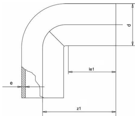
Изгиб ПВДФ 90° (Simona) d75 SDR21 PN16
