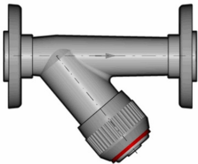
Грязевый фильтр RVOT PBX с фланцевыми окончаниями, EPDM, FIP d40 (DN32)
