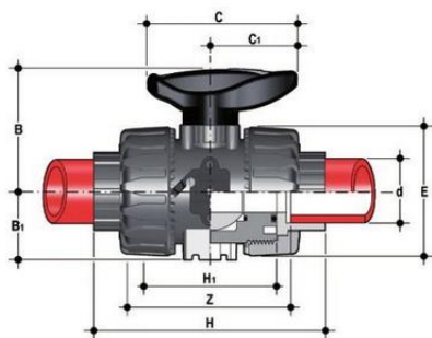
Шаровой кран промышленного применения VKD с муфтовыми окончаниями (уплотнение FKM) PP-H d20 (DN15)
