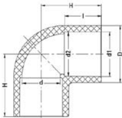
Отвод 90° ХПВХ IPS (Model A) d160 PN16
