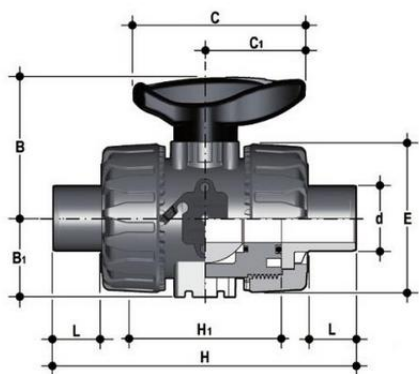
Шаровой кран промышленного применения VKD со втулочными окончаниями (уплотнение EPDM) PP-H d50 (DN40)
