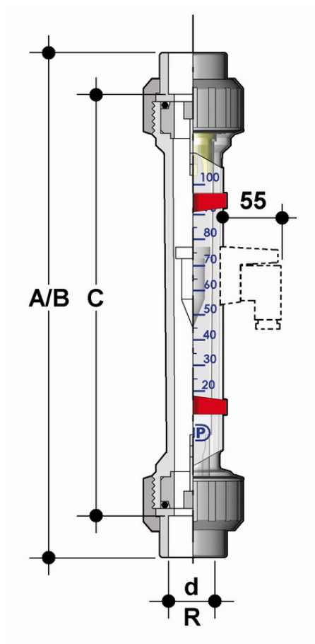
FS ротаметр для воды; корпус: трогамид ; поплавков с магнитом d40
