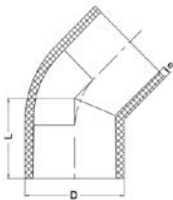
Отвод для стыковой сварки 45° PP-H IPS (Model B) d400 PN10
