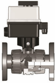
Шаровой кран VKD ПВДФ с эл.приводом 24V AC/DC, фланцевые окончания d50 (DN40)
