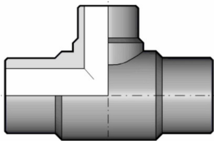
Тройник редукционный для стыковой сварки PP-H FIP (PN10) 63x50 SDR11 PN10
