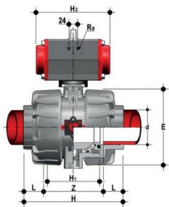
Шаровой кран VKD с пневмоприводом ДвД с муфтовыми окончаниями, DN65-100 (уплотнение EPDM) PP-H d90 (DN80)
