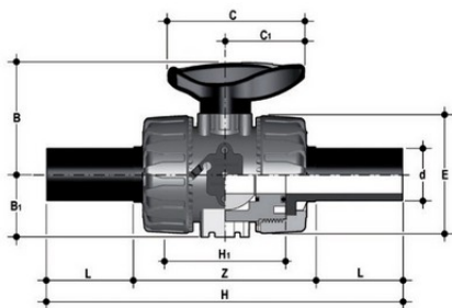
Шаровой кран ПВХ промышленного применения VKD с патрубками из ПЭ (CVDE), FKM, FIP d50 (DN40)
