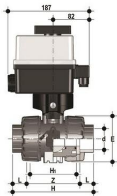
Шаровой кран VKD ХПВХ с эл.приводом 90-240V, муфтовые окончания d32 (DN25)
