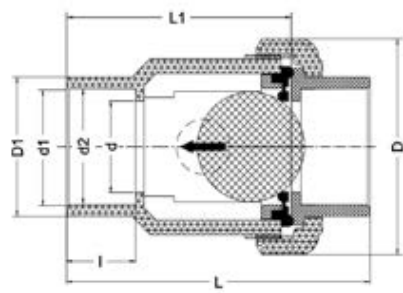
Шаровой обратный клапан с одним разборным окончанием ISR ПВХ; с муфтовыми окончаниям, EPDM, IPS d20 (DN15)
