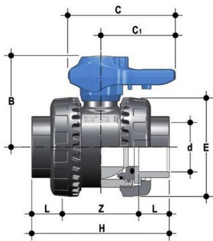
Шаровой кран ПВХ общего применения VEE; муфтовые окончания, EPDM, FIP d32 (DN25)
