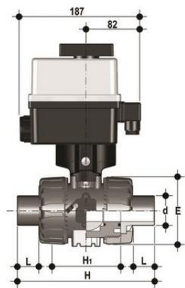
Шаровой кран VKD ПВДФ с эл.приводом 90-240V, втулочные окончания d40 (DN32)
