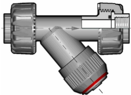
Грязевый фильтр RVUFV PBX с резьбовыми окончаниями, EPDM, FIP R3/8" (DN10)
