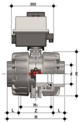
Шаровой кран VKD ПВХ с эл.приводом 24V AC/DC, муфтовые окончания, EPDM, FIP d75 (DN65)
