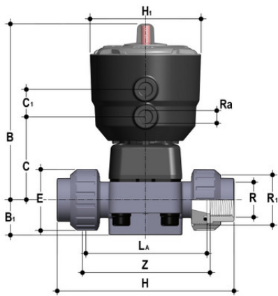
Мембранный клапан ДК ПВХ с пневмоприводом, PN10, резьбовые окончания, EPDM, FIP R3/4" (DN20)
