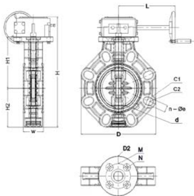
Затвор дисковый промышленный с редуктором ХПВХ IPS (Model A) d12"(DN300)
