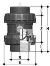
Пружинный шаровой обратный клапан SSE ПБХ; с резьбовыми окончаниями; DN65-100, FKM, FIP R3" (DN80)
